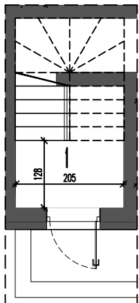
RZUT PARTERU
